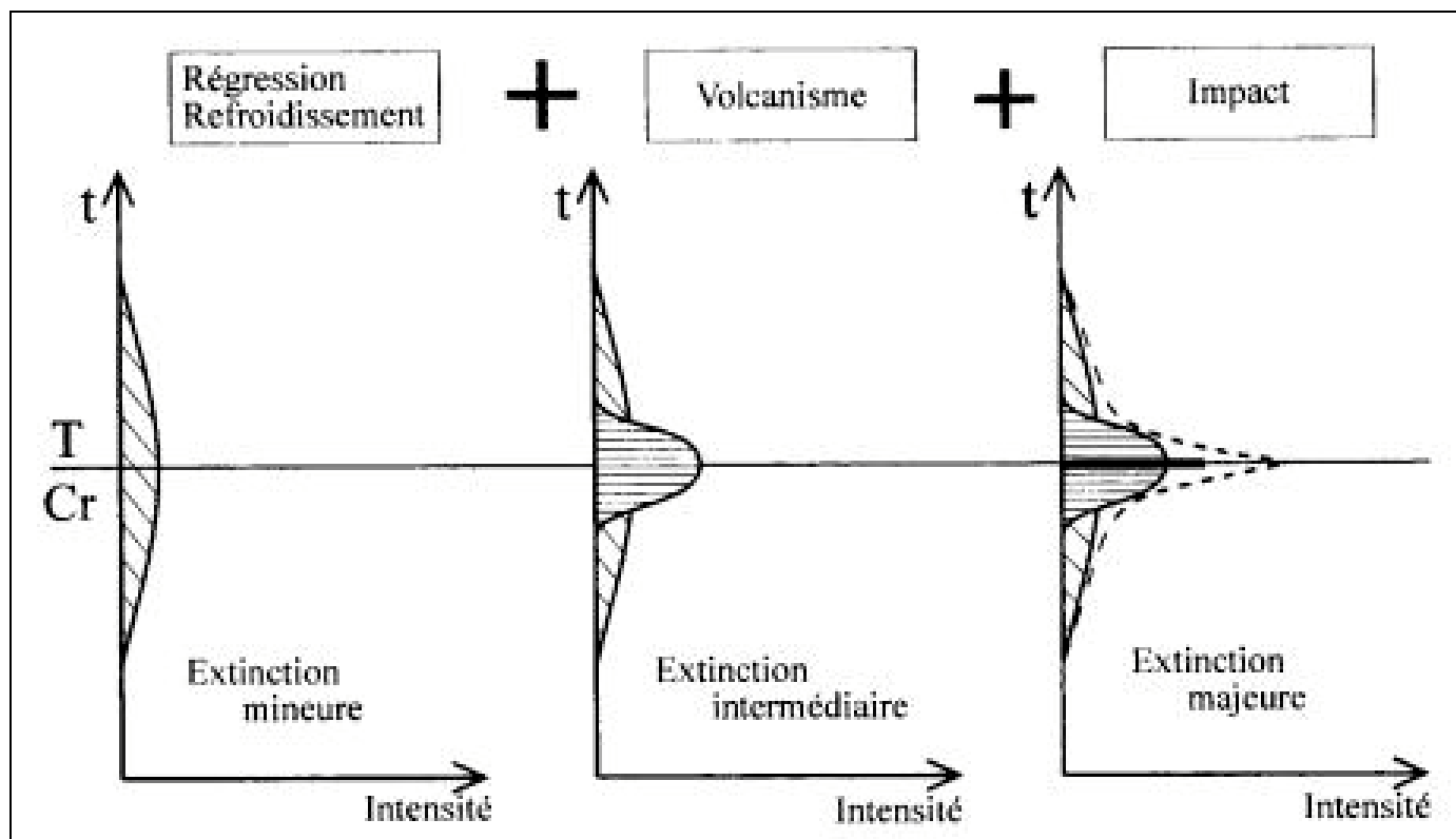
B- Effet cumulé d'évènements géologiques sur les extinctions lors d'une crise biologique
