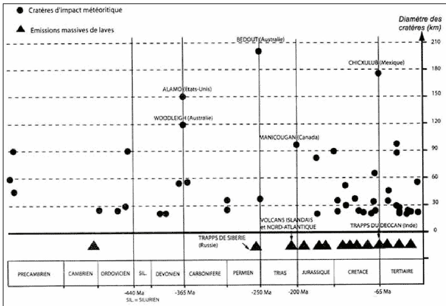
A- Relation entre crises majeures et événements géologiques
