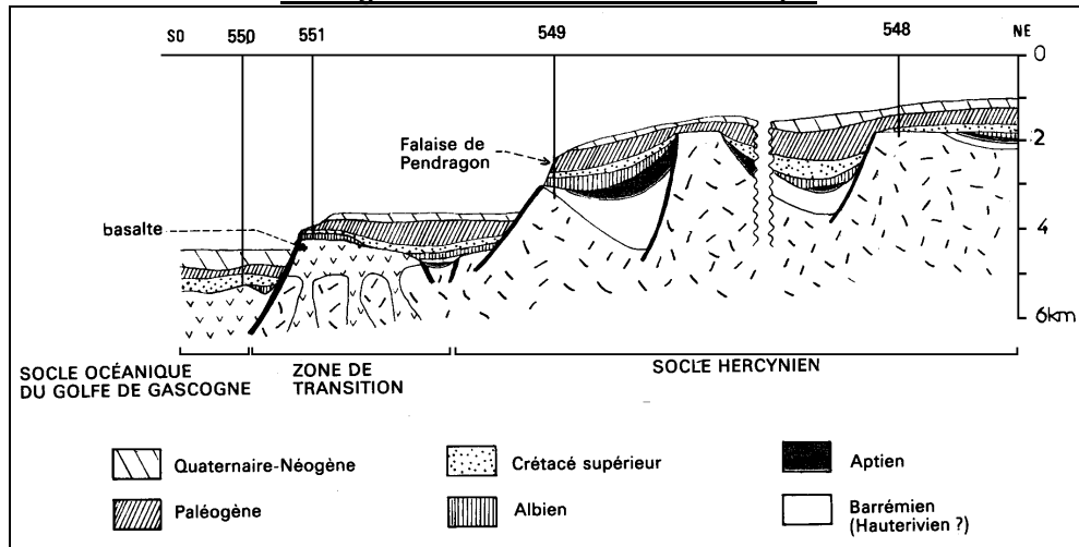
3- Coupe géologique schématique à travers la structure Goban Spur
