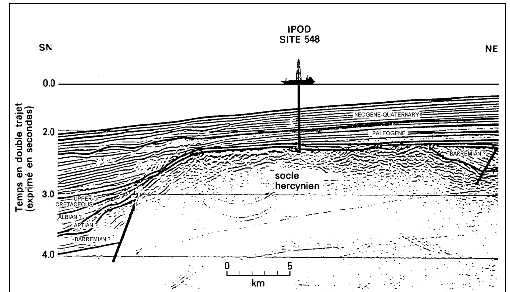
2- Profils sismiques à travers les sites de forage 551 et 548 réalisés au niveau de la structure Goban Spur
