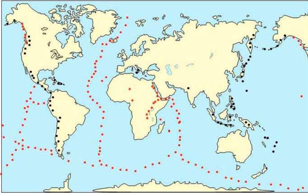
Répartition du volcanisme actif basaltique et andésitique
