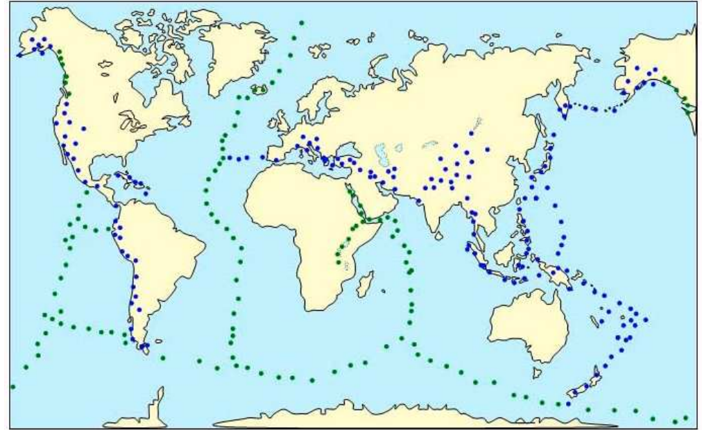
Répartition de la sismicité d'origine extensive et compressive
