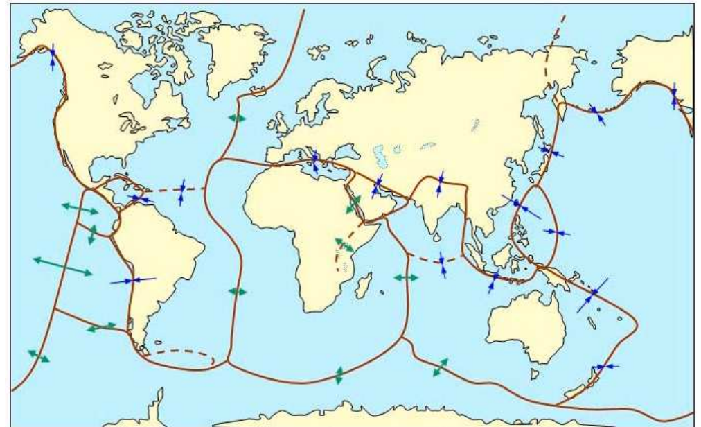
Les mouvements de divergence et de convergence des plaques lithosphériques
