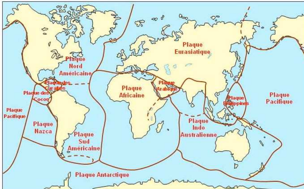
Les principales plaques lithosphériques et leurs limites
